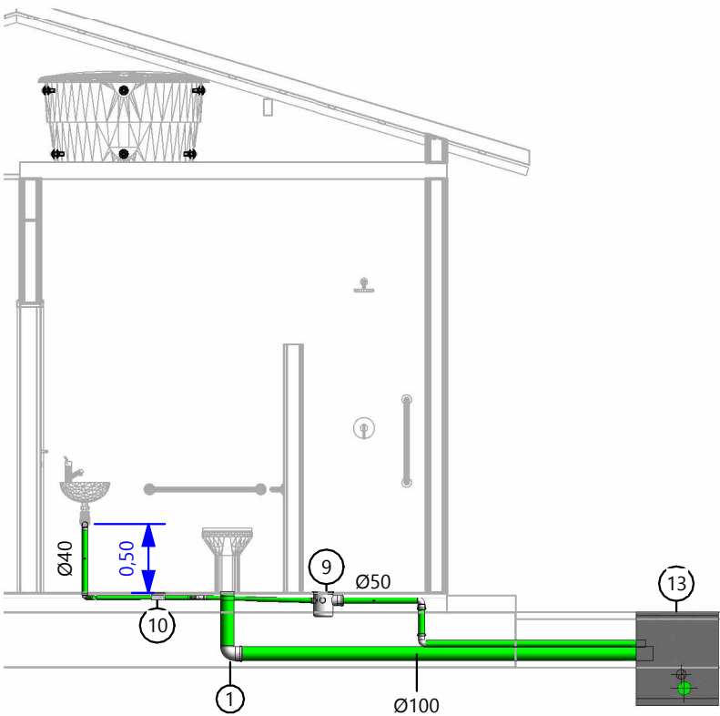
3 I.S. ESC: 1 : 50
