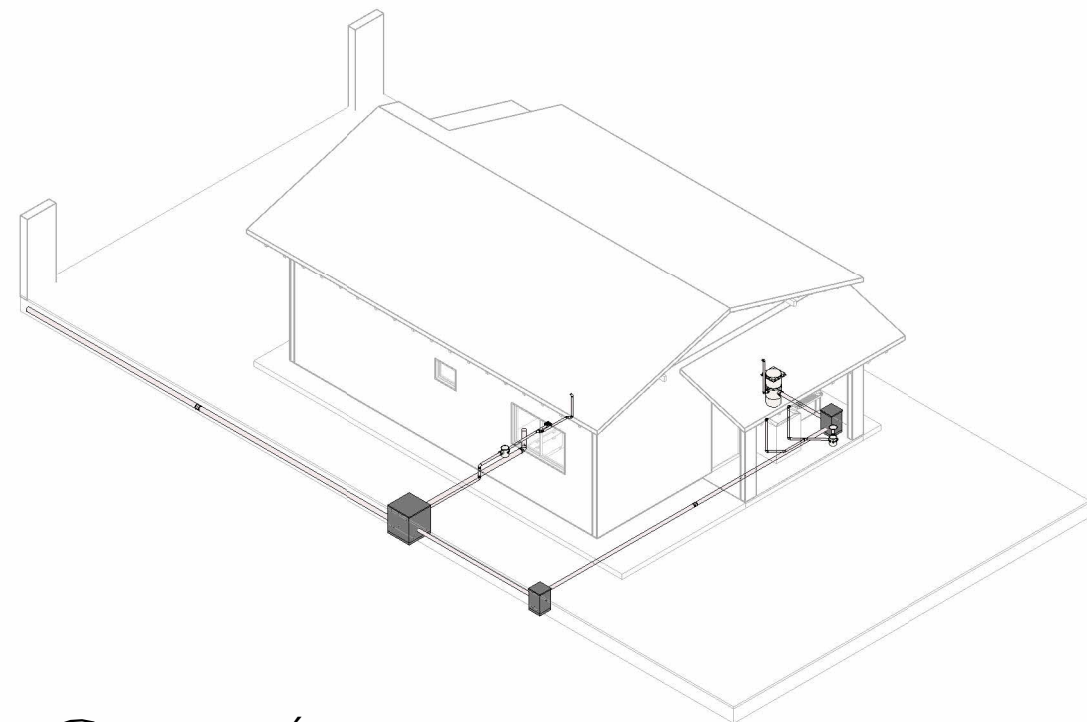
4 ISOMÉTRICO SEM ESCALA
