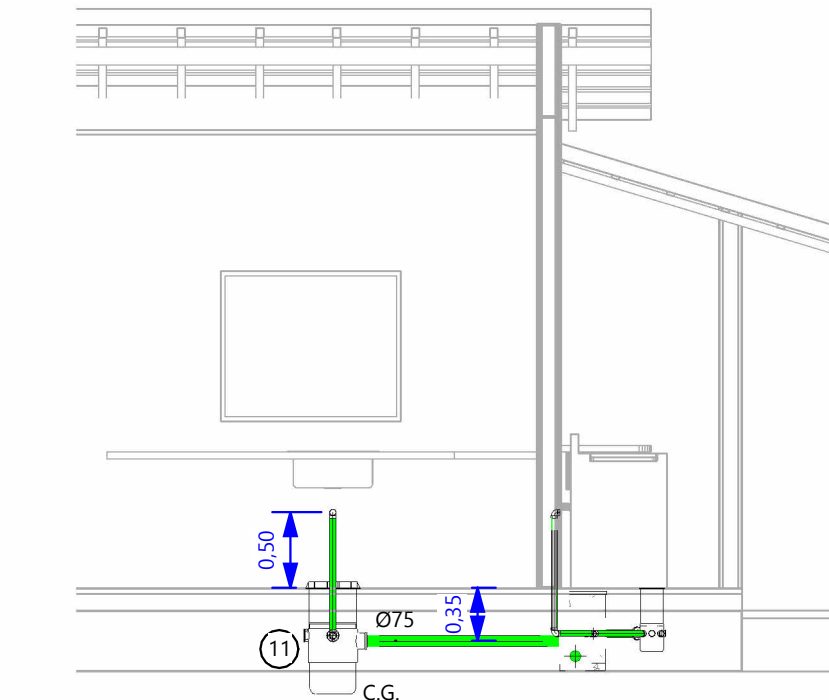
2 COZINHA ESC: 1 : 50
