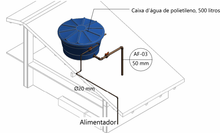
10 DETALHE RESERVATÓRIO SEM ESCALA
