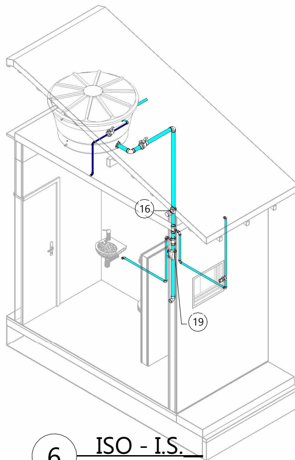
6 ISO - I.S. SEM ESCALA
