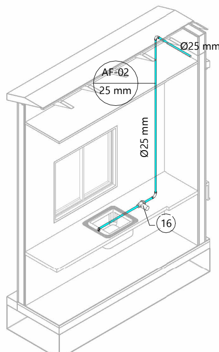
7 ISO - COZINHA SEM ESCALA
