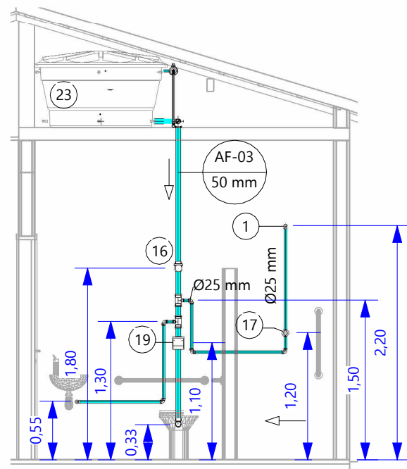
2 DET. I.S. ESC: 1 : 50
