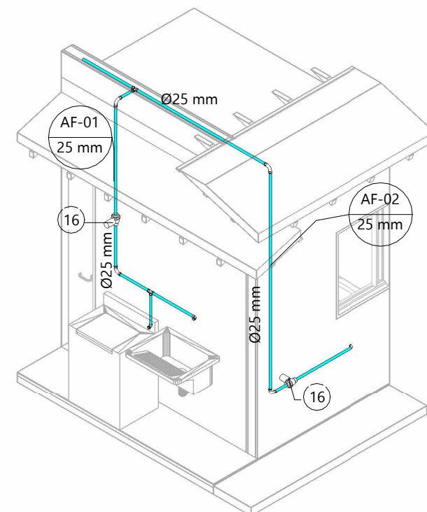
8 ISO - ÁREA DE SERVIÇO SEM ESCALA
