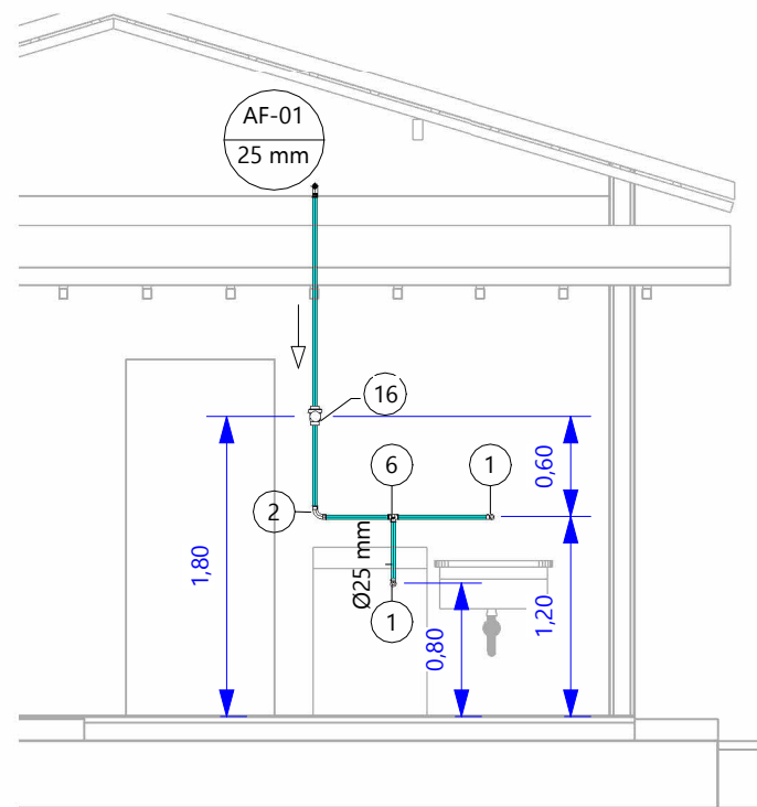
4 DET. Á. SERVIÇO ESC: 1 : 50
