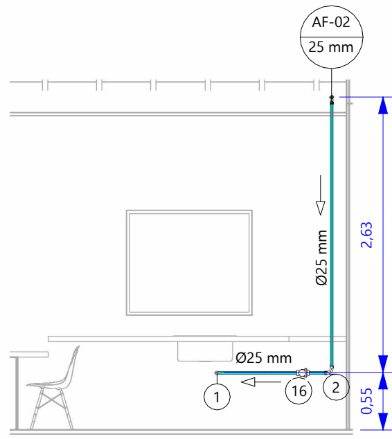
3 DET. COZINHA ESC: 1 : 50
