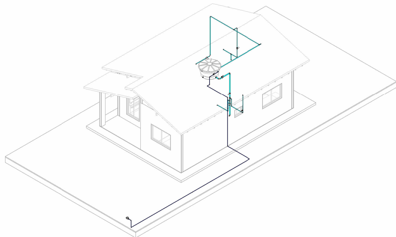
5 PERSPECTIVA SEM ESCALA
