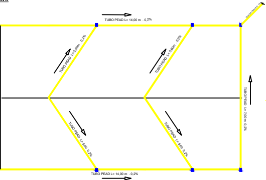
PLANTA SISTEMA DE DRENAGEM Esc. 1:150
