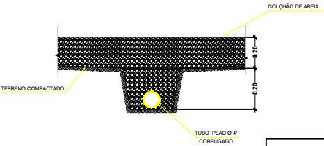
DETALHE SEÇÃO A - A
