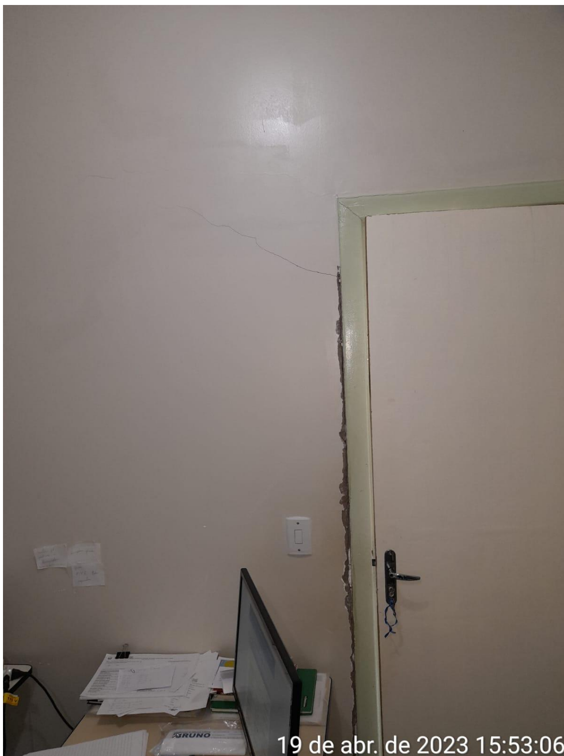
Foto 01 Reparo trinca
