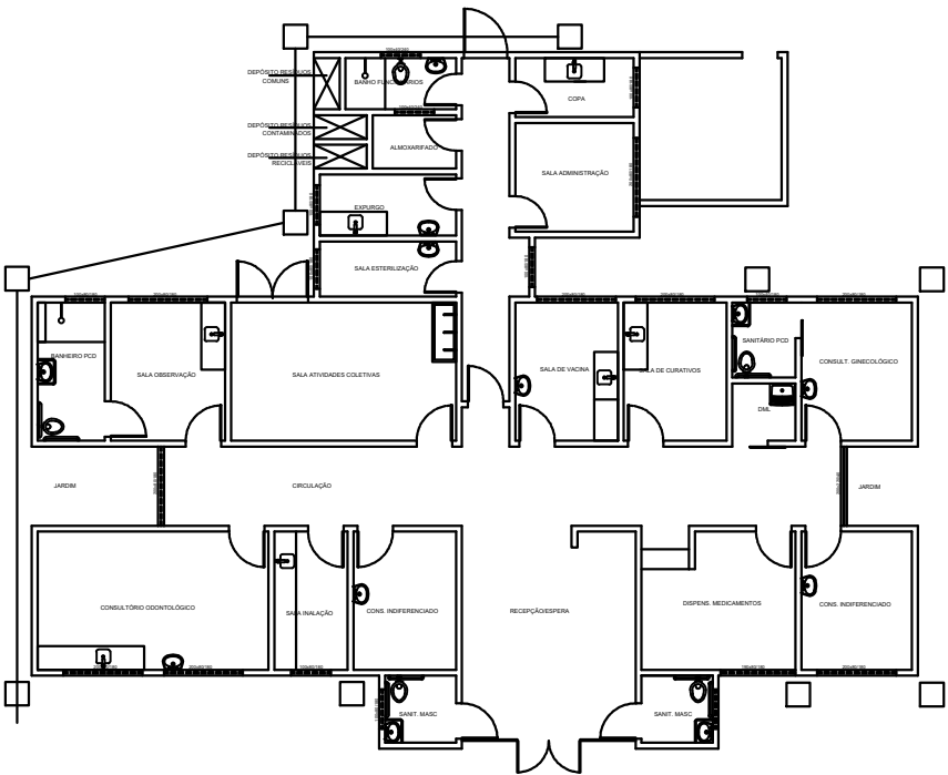
PLANTA BAIXA - LAYOUT ESC.: 1/75
